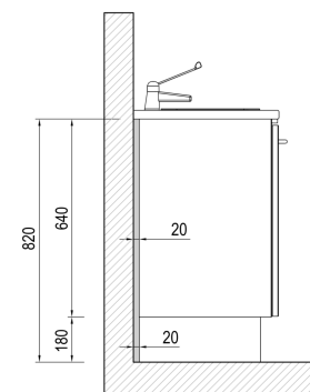
DIMENSIONI DEL VUOTO SANITARIO POSTERIORE, IN VISTA A LATO DEL MOBILE
